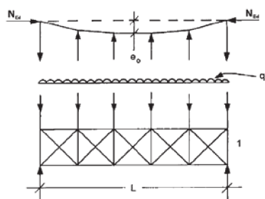
Figura C4.2.5 - Forze equivalenti in sistemi di controvento
