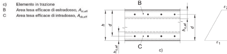
Figura C4.1.10- Area tesa efficace. Casi tipici
