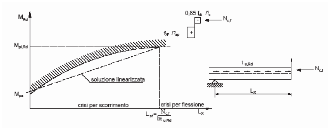
Figura C4.3.9 - Diagramma di interazione parziale calcestruzzo lamiera
