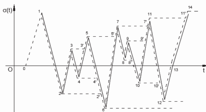
Figura C4.2.20 - Metodo del flusso di pioggia
