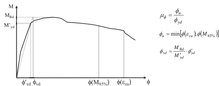
Figura C4.1.12– Relazione momento-curvatura. Fattore di duttilità di curvatura.
