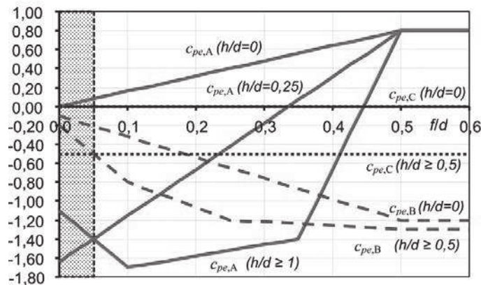
Figura C3.3.27 - Schema di riferimento per cupole sferiche
