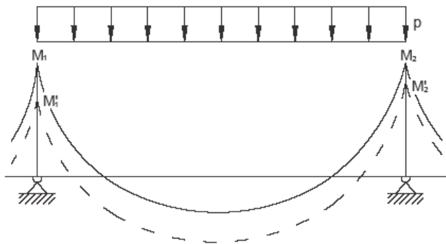
Figura C4.1.1 - Redistribuzione dei momenti per travi continue
