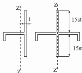
Figura C4.2.12 - Irrigidimenti longitudinali dei pannelli d'anima
