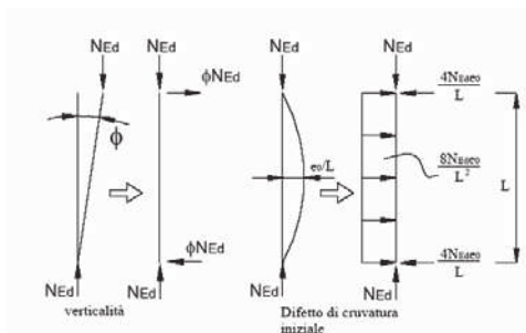
Figura C4.2.4 - Sistemi di forze equivalenti alle imperfezioni
