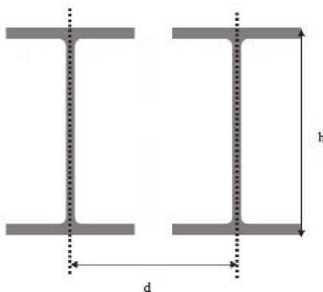
Figura C3.3.28 – Travi parallele
