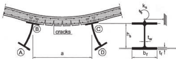
Figura C4.3.7 -Telaio ad U invertita: A-B-C-D
