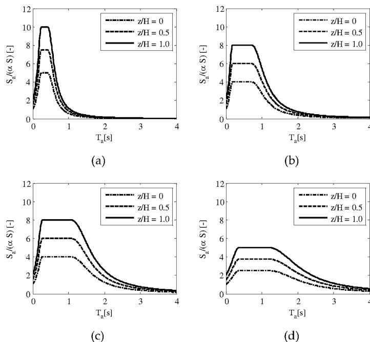
Figura C7.2.4 - Accelerazione massima, normalizzata rispetto ad \alpha S , per i seguenti valori di T_1 : (a) T_1 = 0,3 s, (b) T_1 = 0,6 s, (c) T_1 = 0,9 s, (d) T_1 = 1,2 s.
