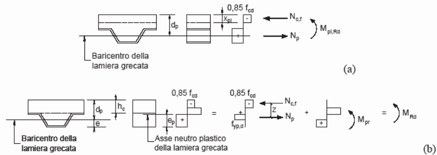
Figura C4.3.8 - Distribuzione plastica delle tensioni: (a) asse neutro nel calcestruzzo sopra la lamiera; (b) asse neutro che taglia la lamiera grecata
