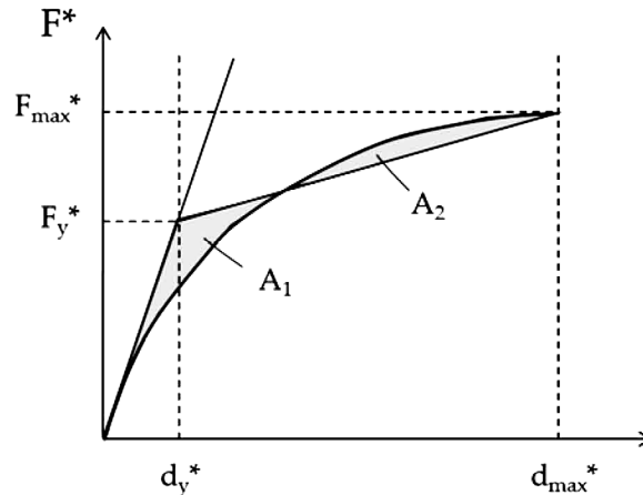
Figura C7.3.3– Bilinearizzazione equivalente
