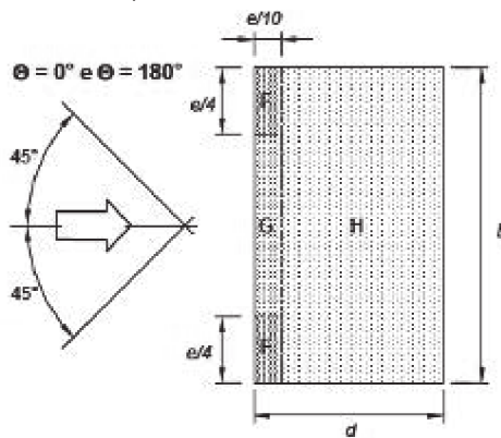
Vento ortogonale alla direzione del colmo
