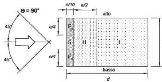
Vento parallelo alla direzione del colmo
