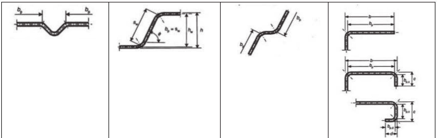
Figura C4.2.27 -Esempi di determinazione della larghezza b_p
