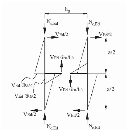
Figura C4.2.9 -Schema di calcolo semplificato per un'asta calastrellata
