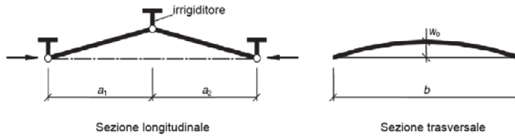
Figura C4.2.18 - Schema di calcolo per gli irrigiditori trasversali
