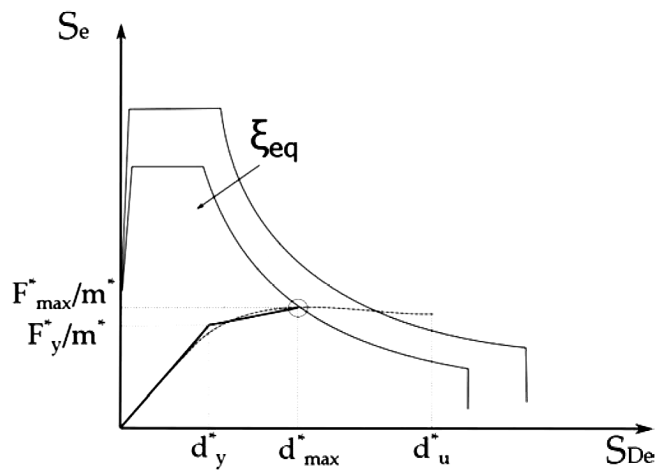
Figura C7.3.4– Individuazione del Punto di prestazione
